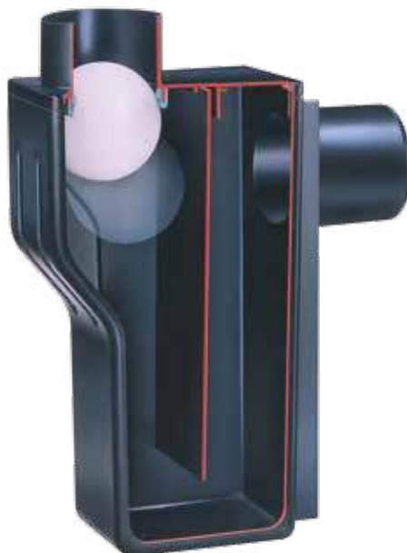
mit Kanal-Rückstausicherung ohne Kleintierschutz
