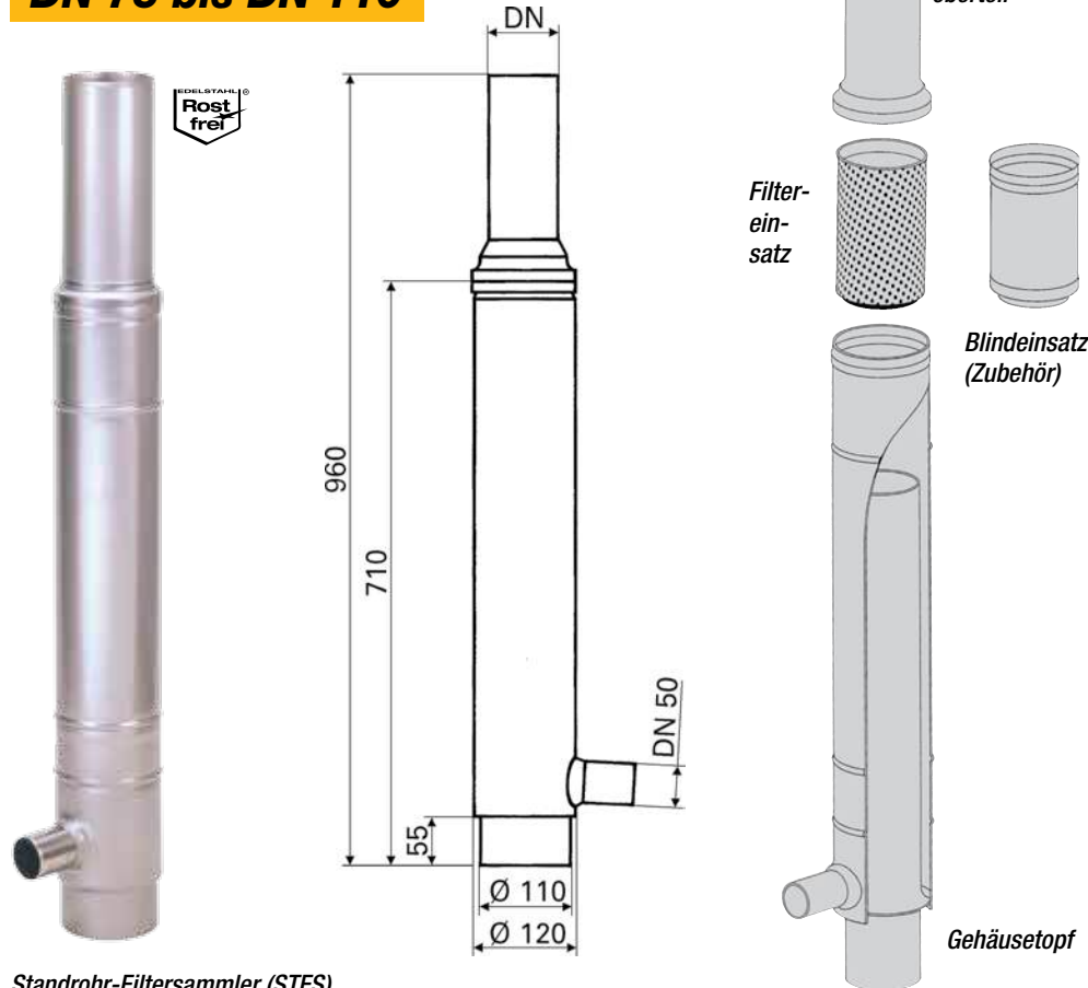
Standrohr-Filter Sammler (STFS)
