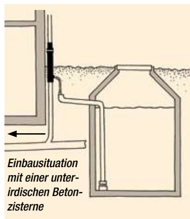
Standrohr-Filter Sammler (STFS)
