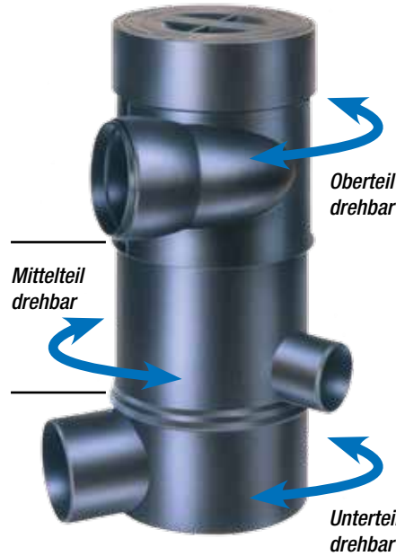
WFF 150 ohne Verlängerungsrohr
