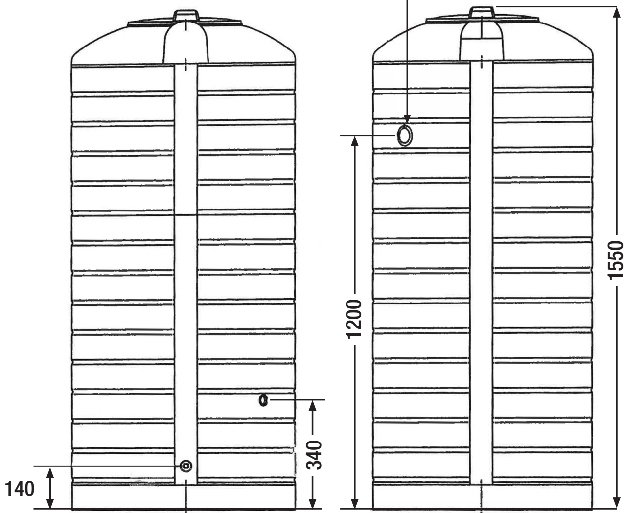
Regensammelereinlauf
