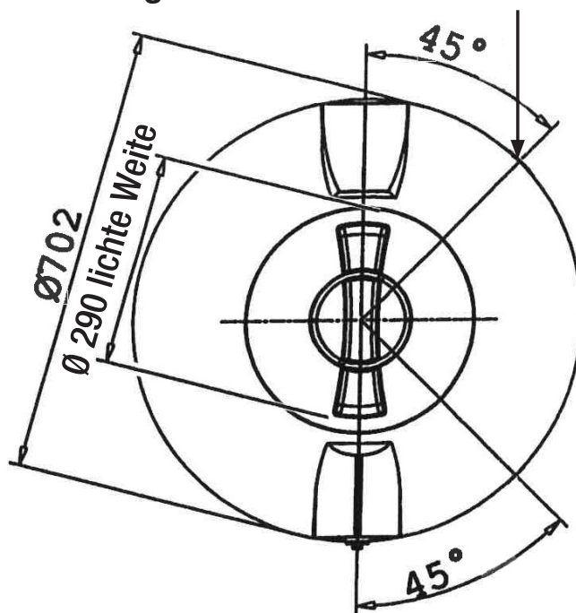
Regensammelereinlauf mit Dichtung für Einlaufstutzen 1¼
