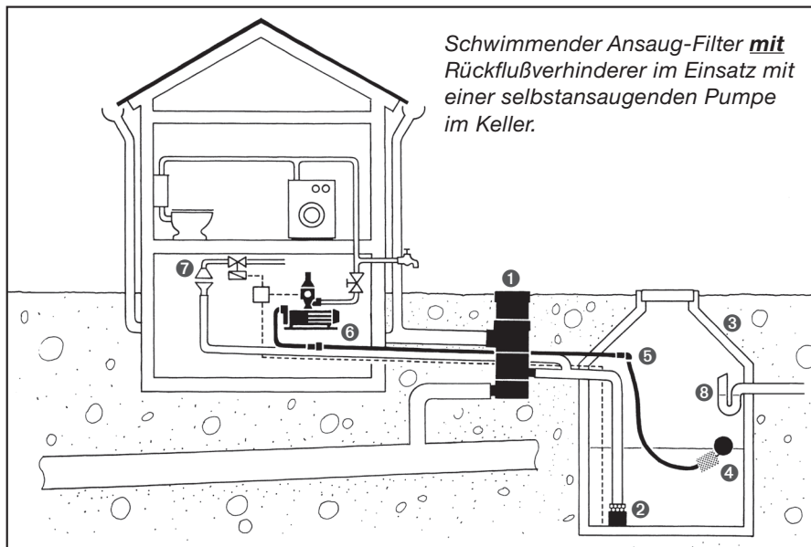
Prinzipische Skizze (Abb. 1) Anlage mit einer Saugpumpe im Keller.
