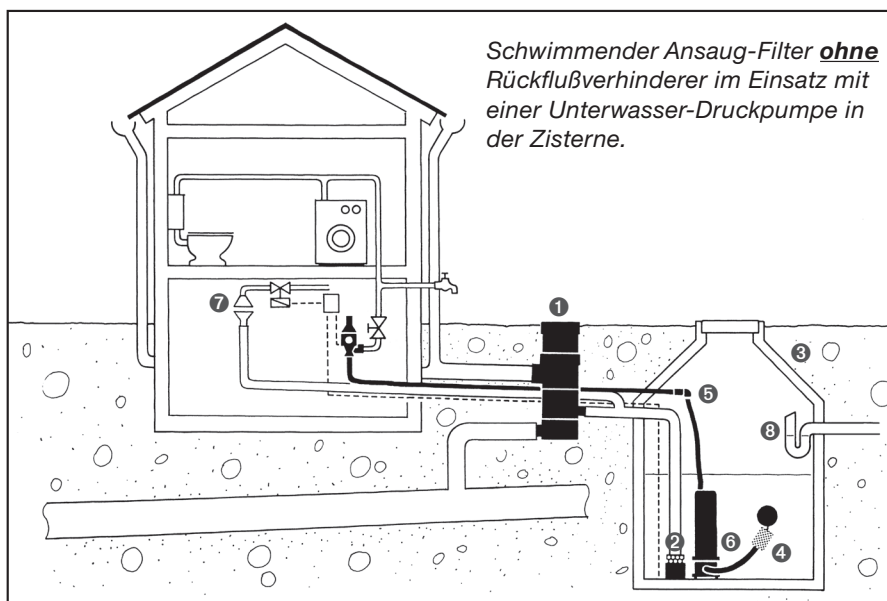
Prinzipische Skizze (Abb. 2) Anlage mit einer Druckpumpe in der Zisterne.
